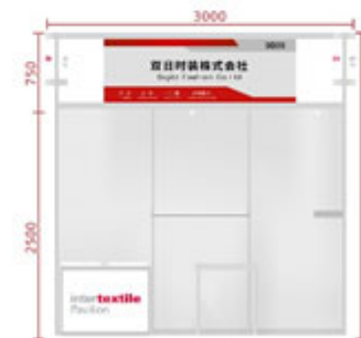
立面図 単位：mm（毫米）
